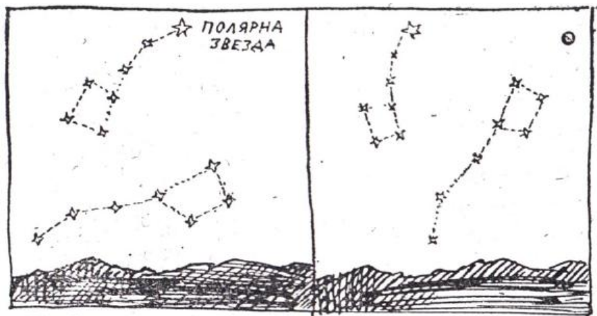
СЪЗВЕЗДИЯТА ГОЛЯМА И МАЛКА МЕЧКА СЛЕДСТВИЕ ДЕНОНОЩНОТО ВЪРТЕНИЕ НА НЕБЕСНАТА СФЕРА, ВИДИМО ОБИКАЛЯТ ОКОЛО СЕВЕРНИЯ НЕБ. ПОЛЮС
