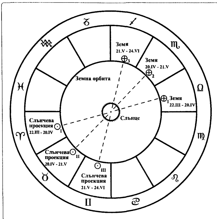
Фигура 8. Хелиоцентрична и геоцентрична гледна точка.
