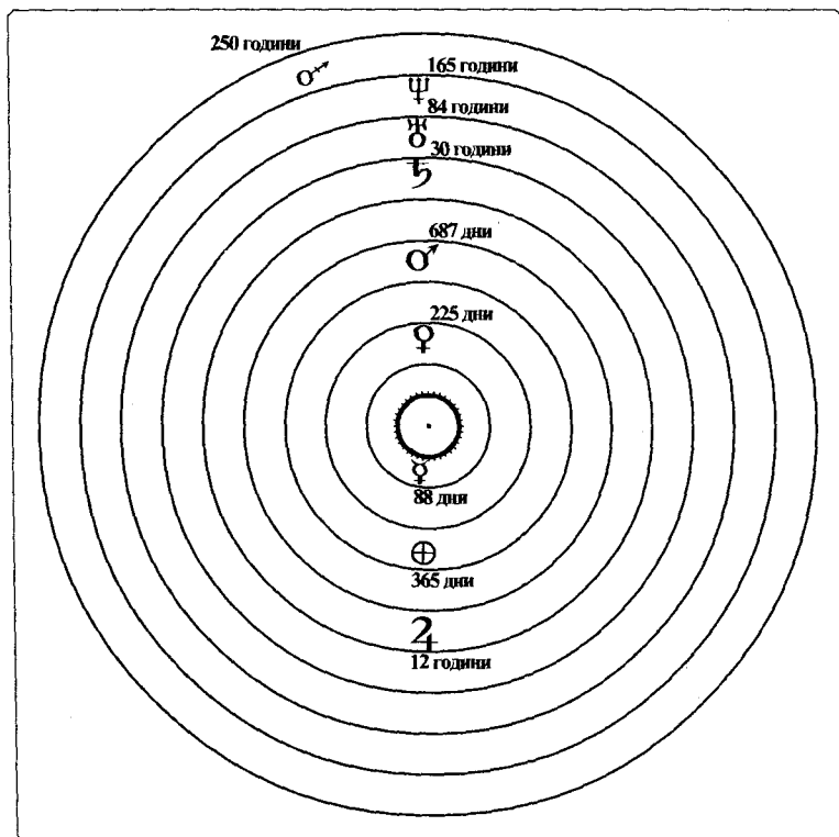
Фигура 9. Орбити на планетите от Слънчевата система.
